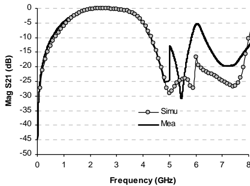
Fig.8. Scattering parameters
